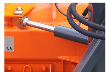
Hydraulische Seitenverstellung
